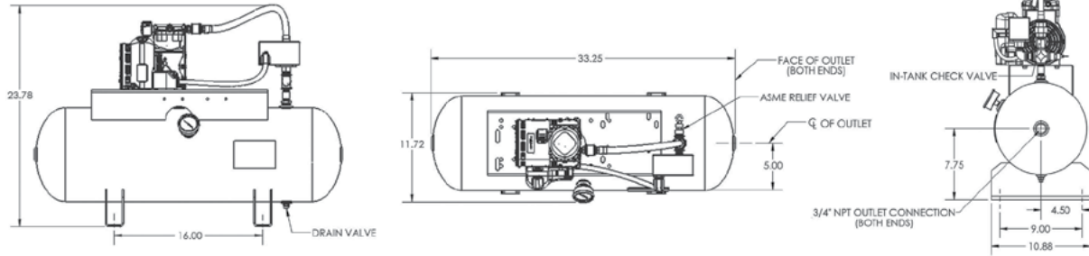
MODEL: OLT120-A
