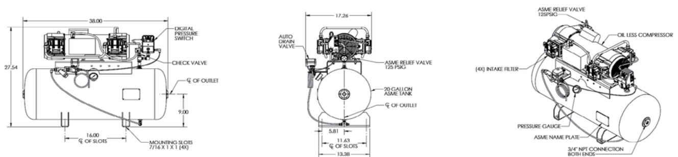
MODELS: OLTV915-A | OLTV1095-A
