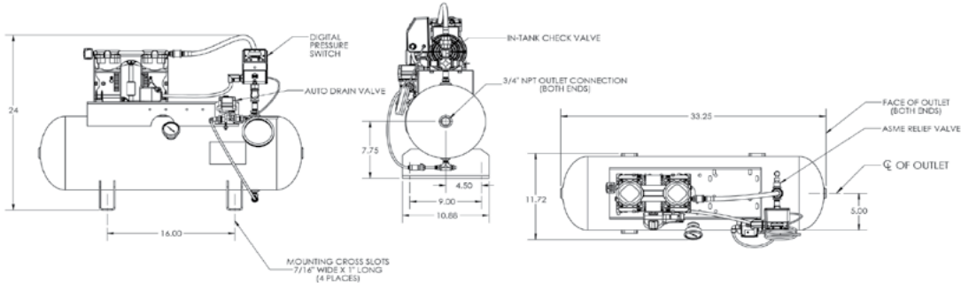
MODELS: OLTV400-A | OLTV500-A | OLTV600-A
